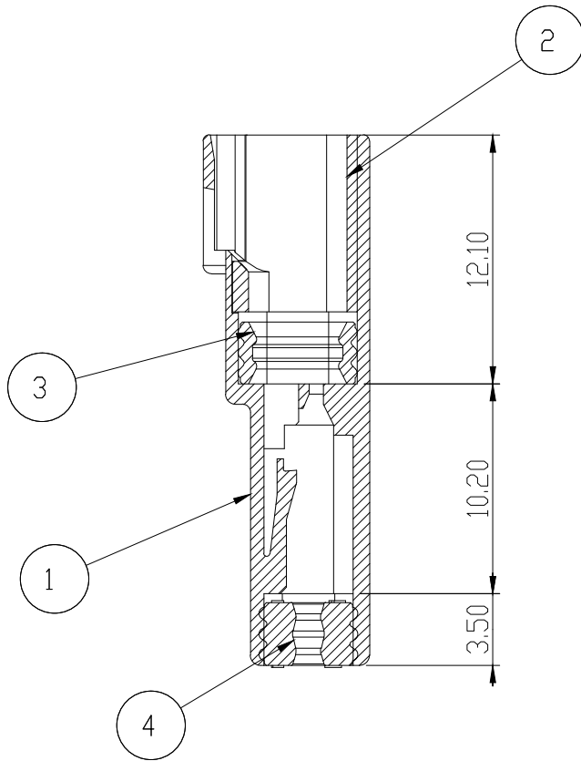
단면 A-A
