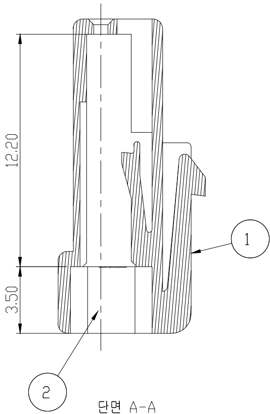
단면 A-A
