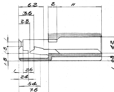
"B" 部 DETAIL
