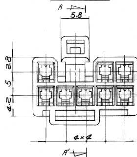
"B" 部 DETAIL
