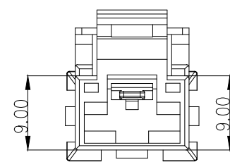
A-TYPE (P/NO.:MG615575)
