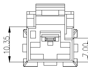
C-TYPE (P/NO.:MG613689)
