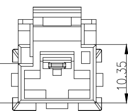
B-TYPE (P/NO.:MG610658)
