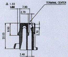
SEC. A-A
