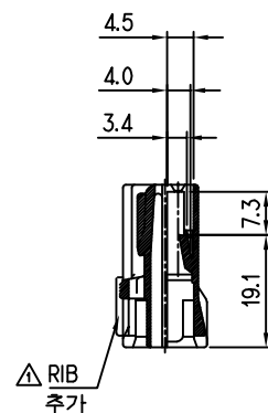
SEC. A-A
