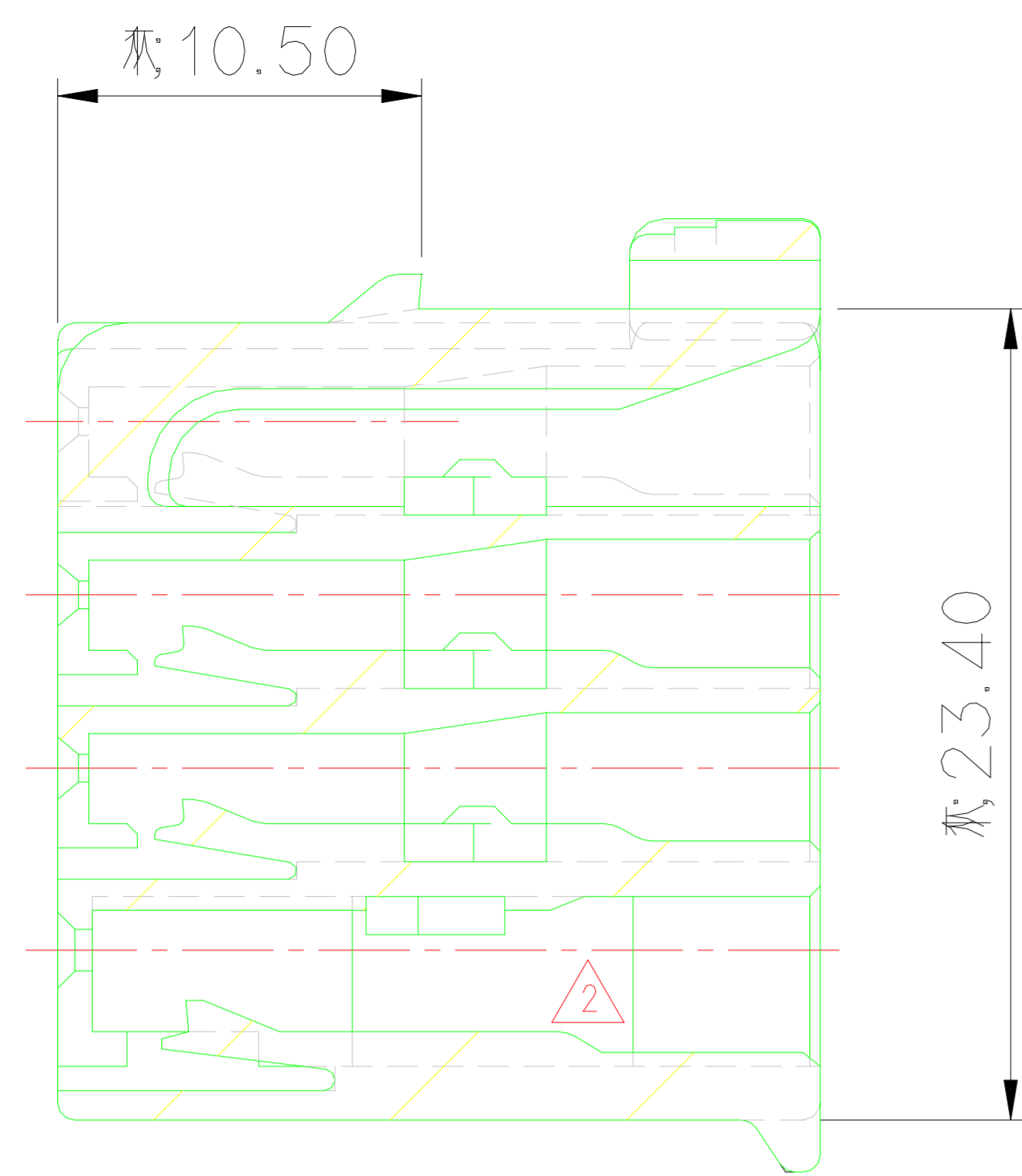
SECTION A-A
