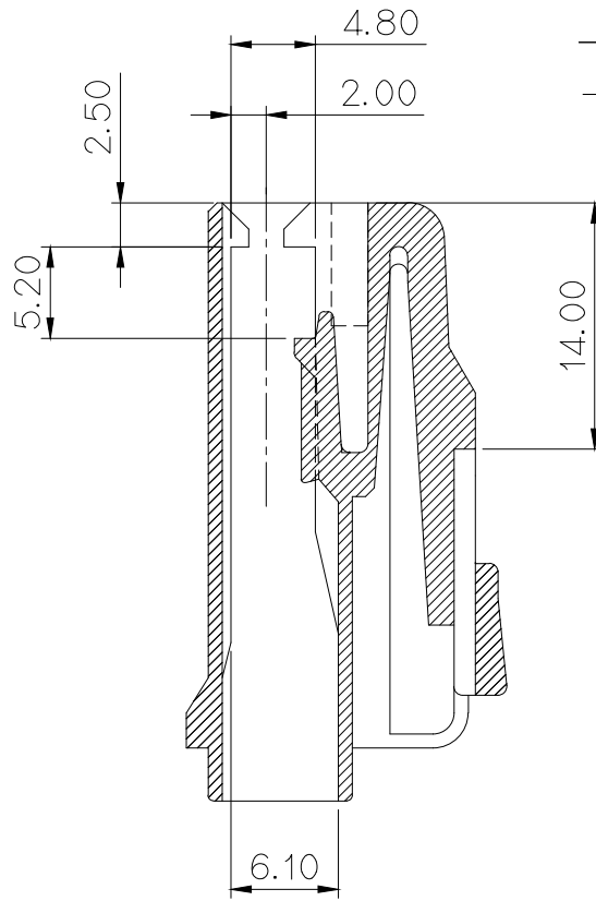
SECTION A-A
