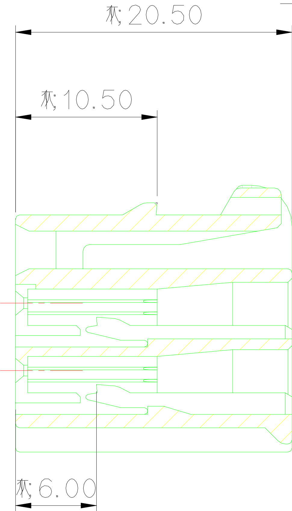
SECTION A-A
