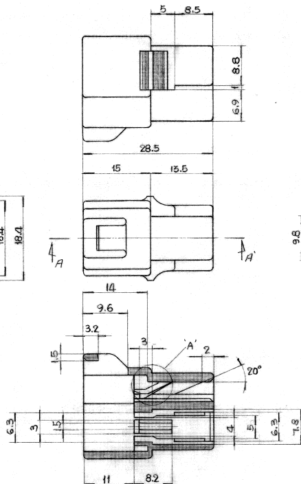
SECTION A-A'
