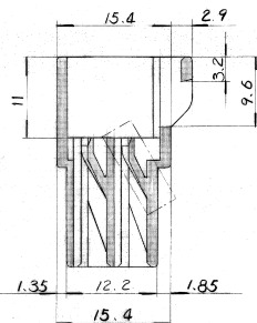
LOCK 부 상세도
