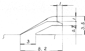
LOCK 부 상세도
