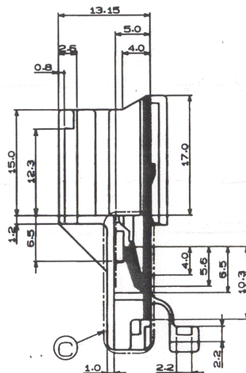
SEC. A-A
