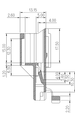
SEC. A-A
