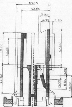
SEC. A-A
