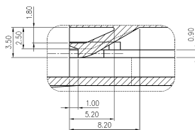
DETAIL 'C,(S:5/1)
