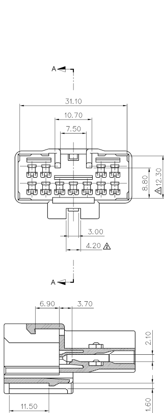
SECTION A-A
