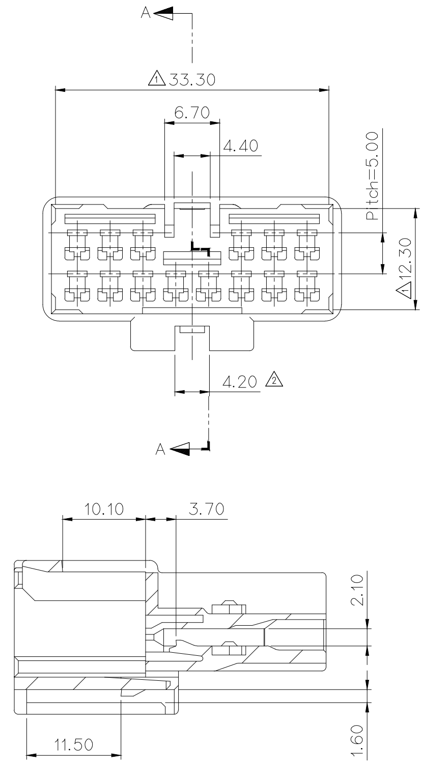
SECTION A-A
