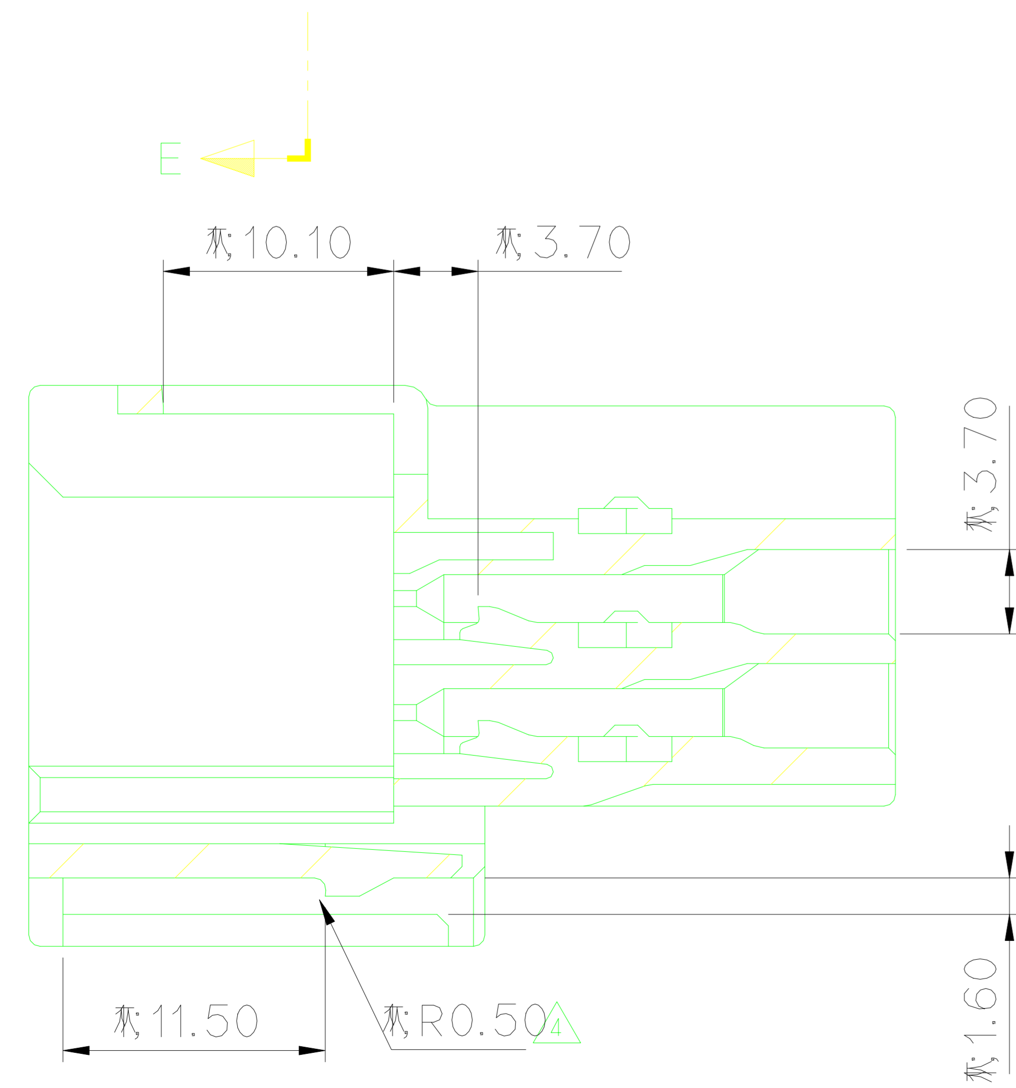
SECTION A-A
