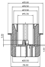
SEC. A-A
