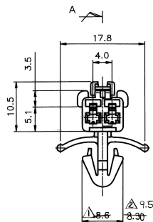
적용 BRACKET 형상 (2/1)
