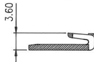
SEC. A-A
