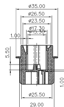
SEC. A-A
