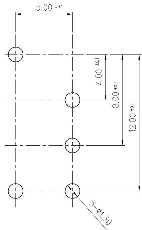
DIM. OF PCB
