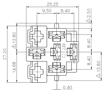
SEC A-A
