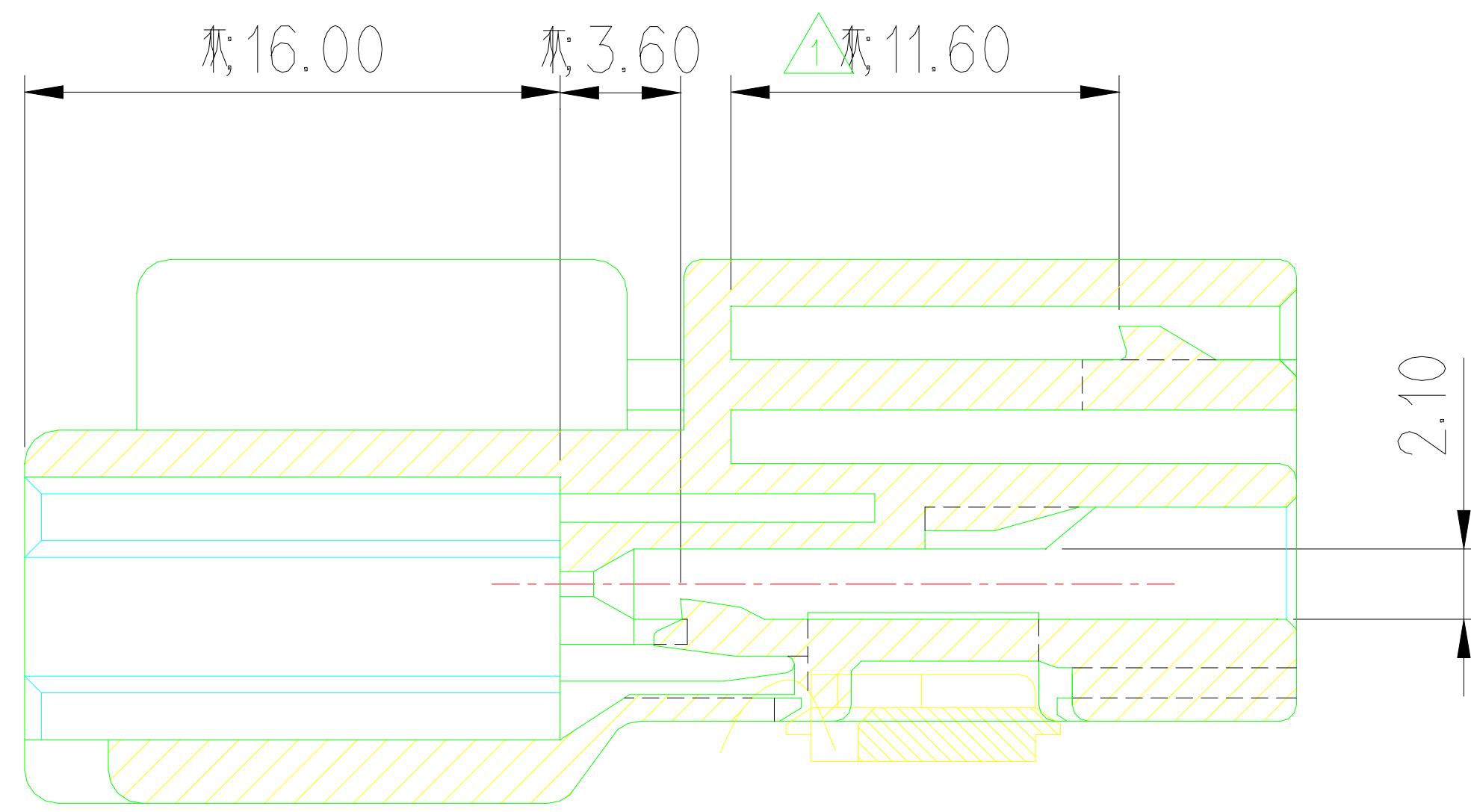
SECT 9 A-A
