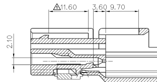
SECT' A-A
