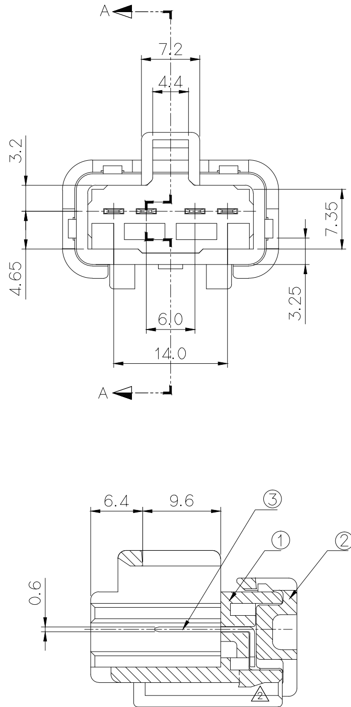
SECTION A-A
