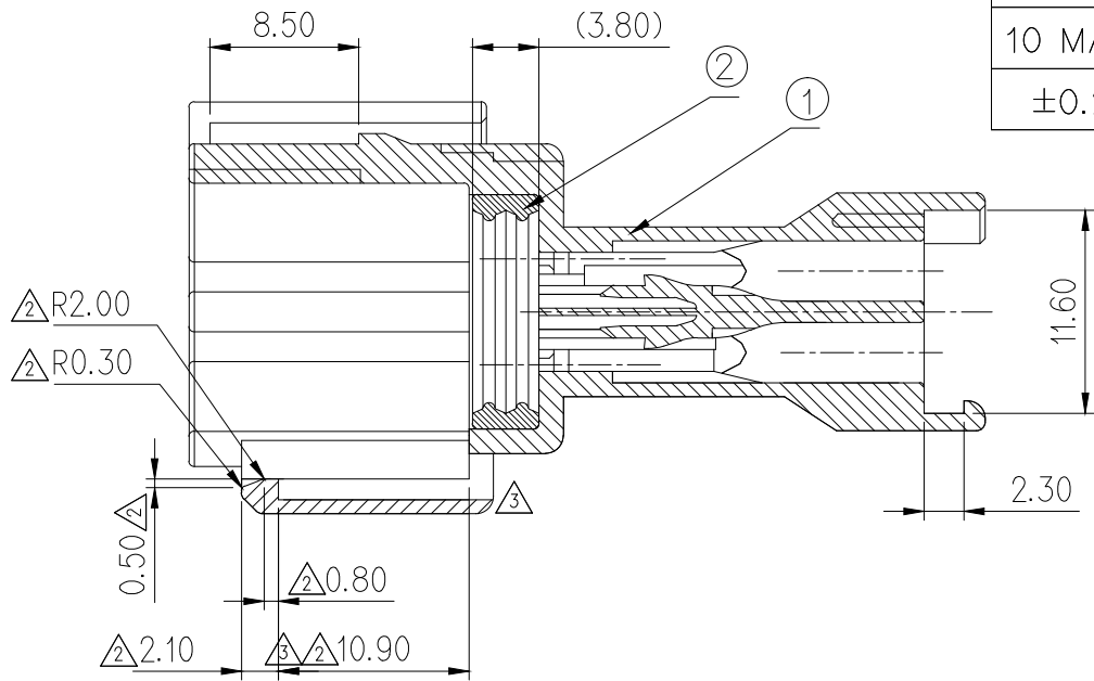
SECTION A-A'
