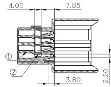
SECTION A-A ( 040 )
