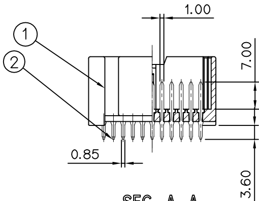
SEC. A-A
