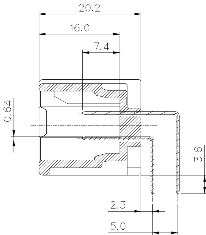
SECTION A-A
