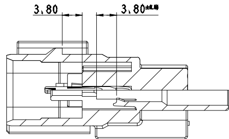
SECTION B-B(FAKRA)
