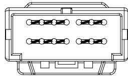
4+3+4+3 JOINT-CIRCUIT MG646292-2
