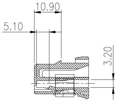
SECT' A-A
