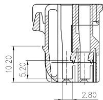
SECT' A-A
