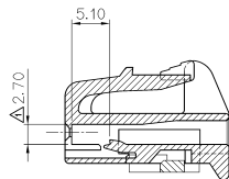
SEC. A-A
