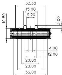
JOINT-CIRCUIT (MG652040-1)
