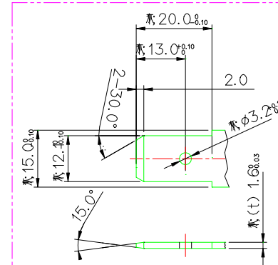
BRACKET 사양
