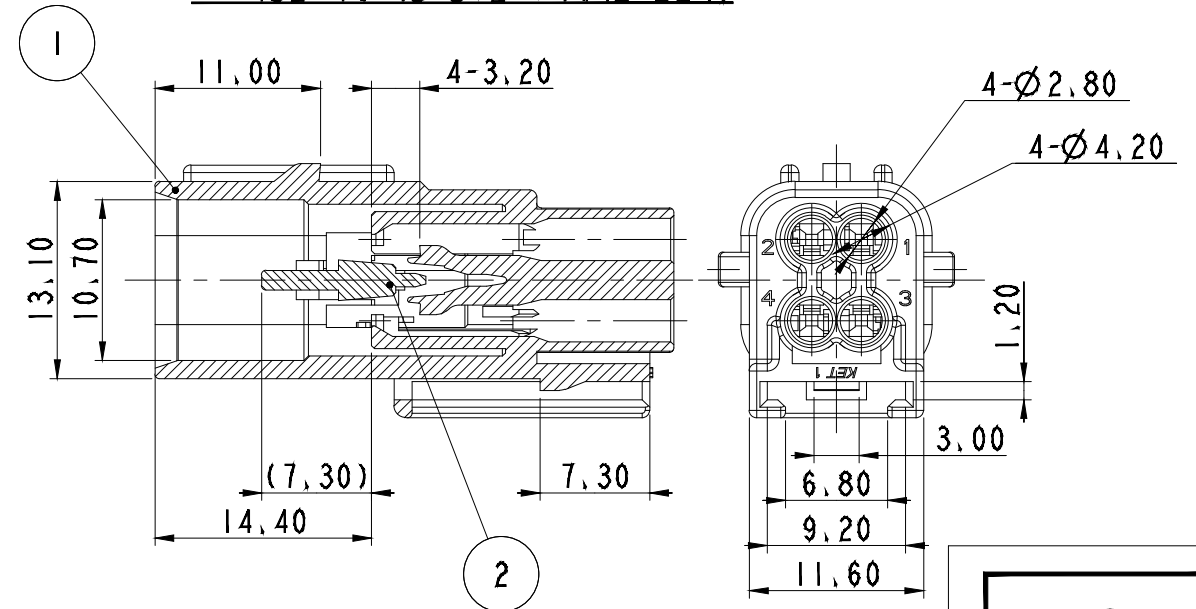
SECTION A-A
