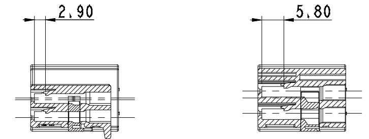
SECTION B-B(060) SECTION C-C(110)
