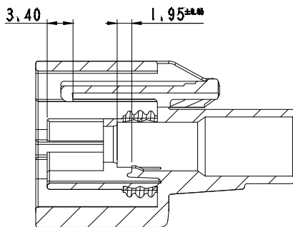
SECTION B-B(FAKRA)
