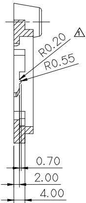
SECTION A-A
