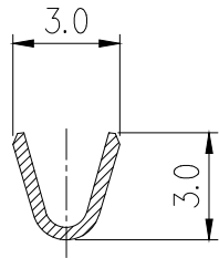
SECTION 'B'
