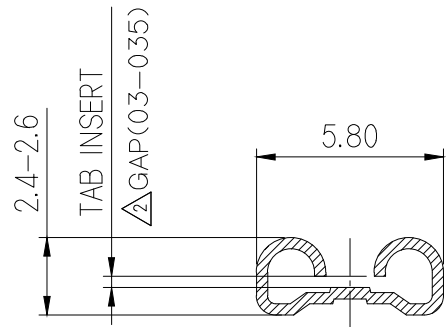
SECTION 'A'
