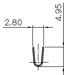
SEC A-A
